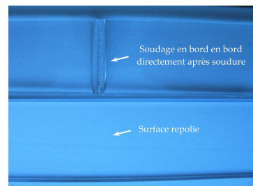
Soudage en bord à bord de PMMA.
