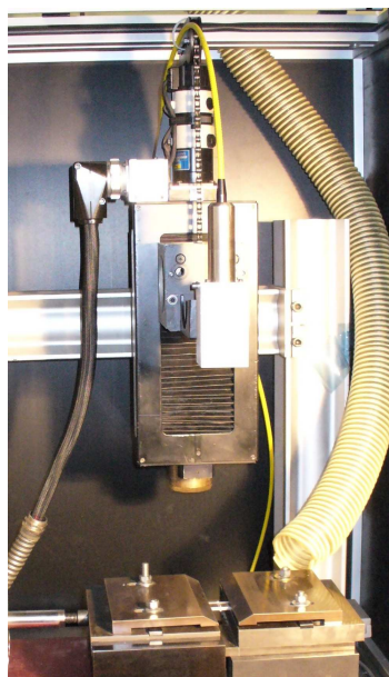
Station d'assemblage d'éléments thermoplastiques en bord à bord à l'aide d'un laser émettant à 1,9 \mu\text{m} .
