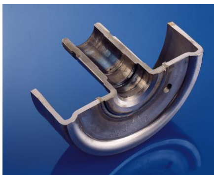
Soudage laser métallique d'organes mécaniques
